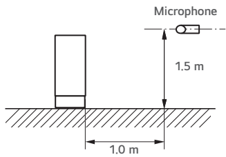
Compressor Module
